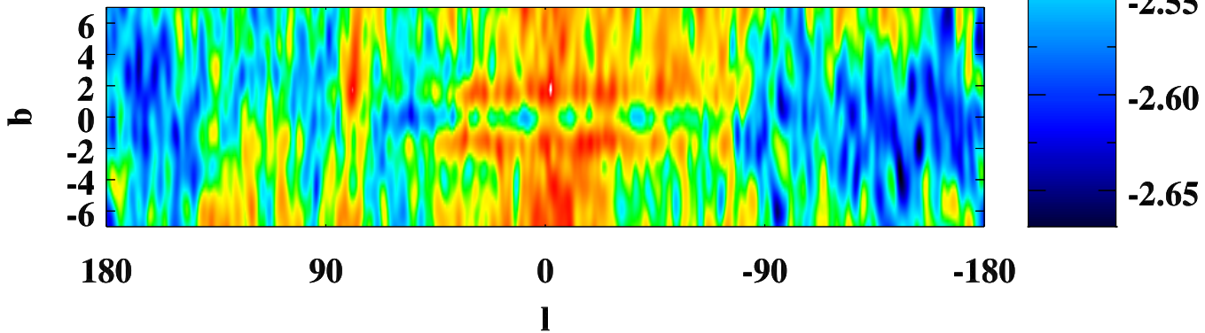
Spectral index 0.85-6.79 GeV: Fermi Data
